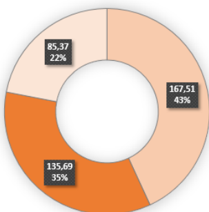
Struktura PO4
