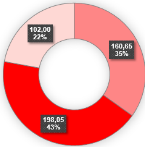
Struktura PO3
