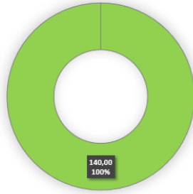
Struktura PO2
