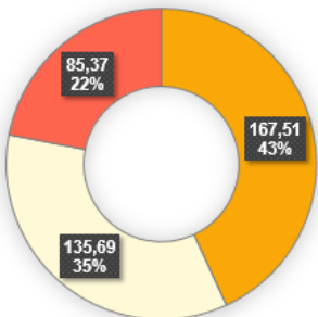
Struktura PO4
